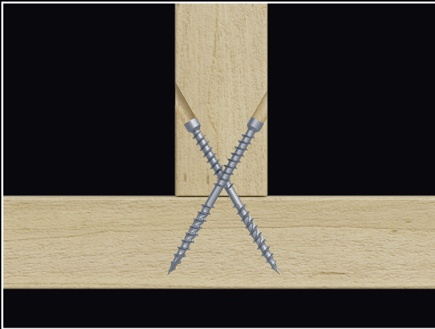
Regelskarv
