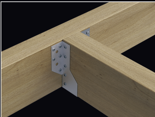
Traditionella beslag
