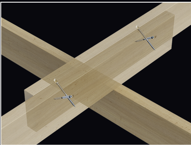
Takstolsinfästning
