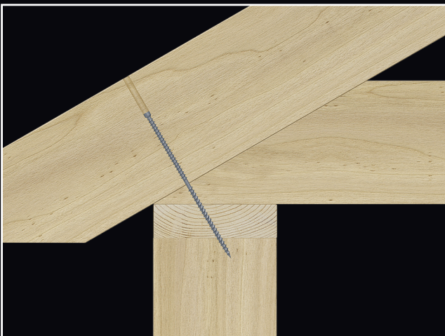
Takstolsinfästning
