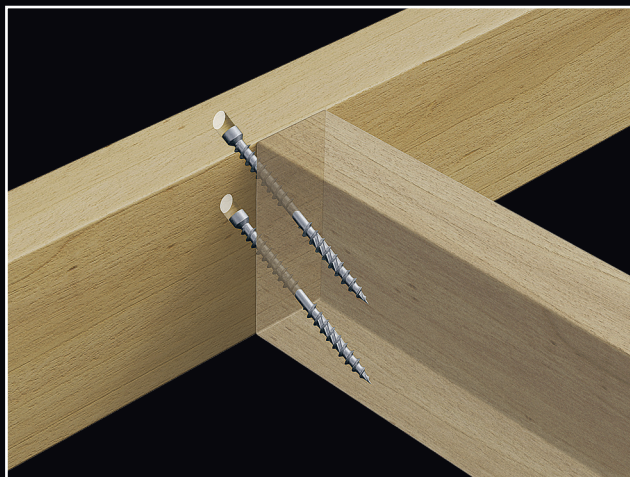
Konstruktionsskruv Jetting
